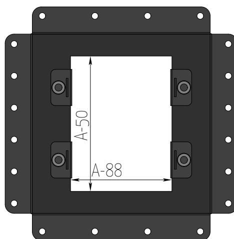
Корпус
